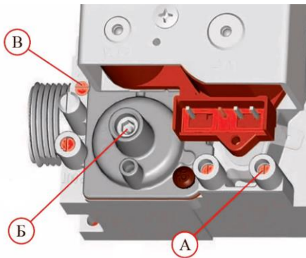
Рис. 16. Газовый клапан Sit 848 Sigma
