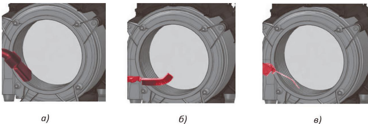
Рис. 18. Чистка камеры сгорания
