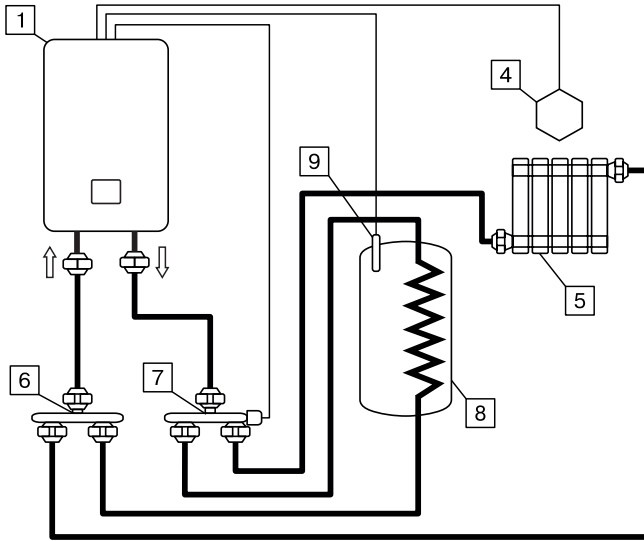
Рис.5 Упрощённая схема подключения миникотельной в режиме «Отопление-ГВС».
