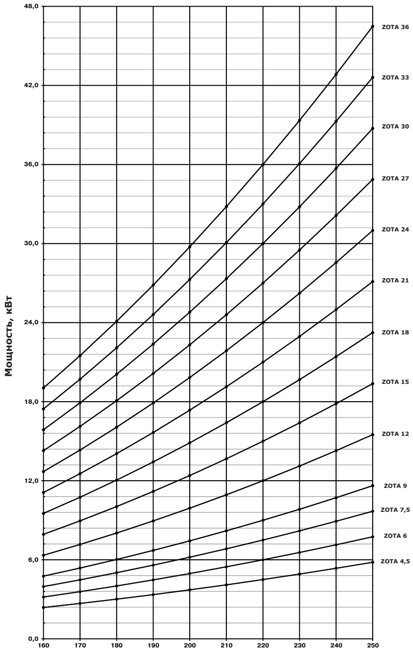
Рис.7 График изменения мощности миникотельной в зависимости от питающего напряжения.
