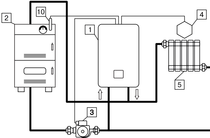
Рис.6 Упрощенная схема подключения миникотельной в режиме вспомогательной.
